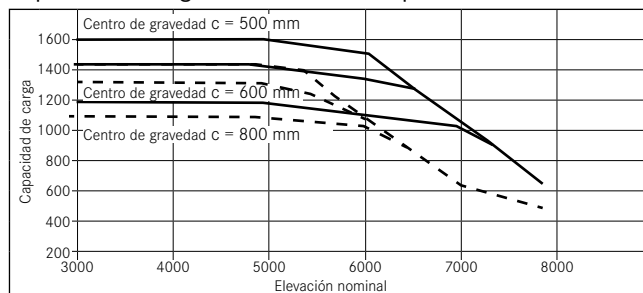
Capacidad de carga RX 60-16 Mástil triple
