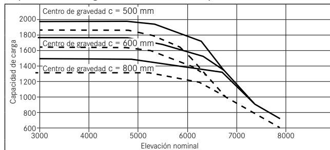
Capacidad de carga RX 60-20 Mástil triple
