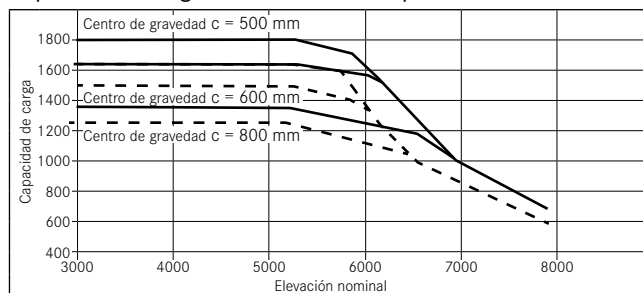
Capacidad de carga RX 60-18 Mástil triple
